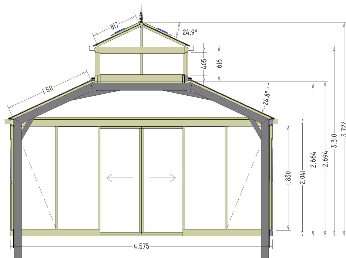
SCHNITT
