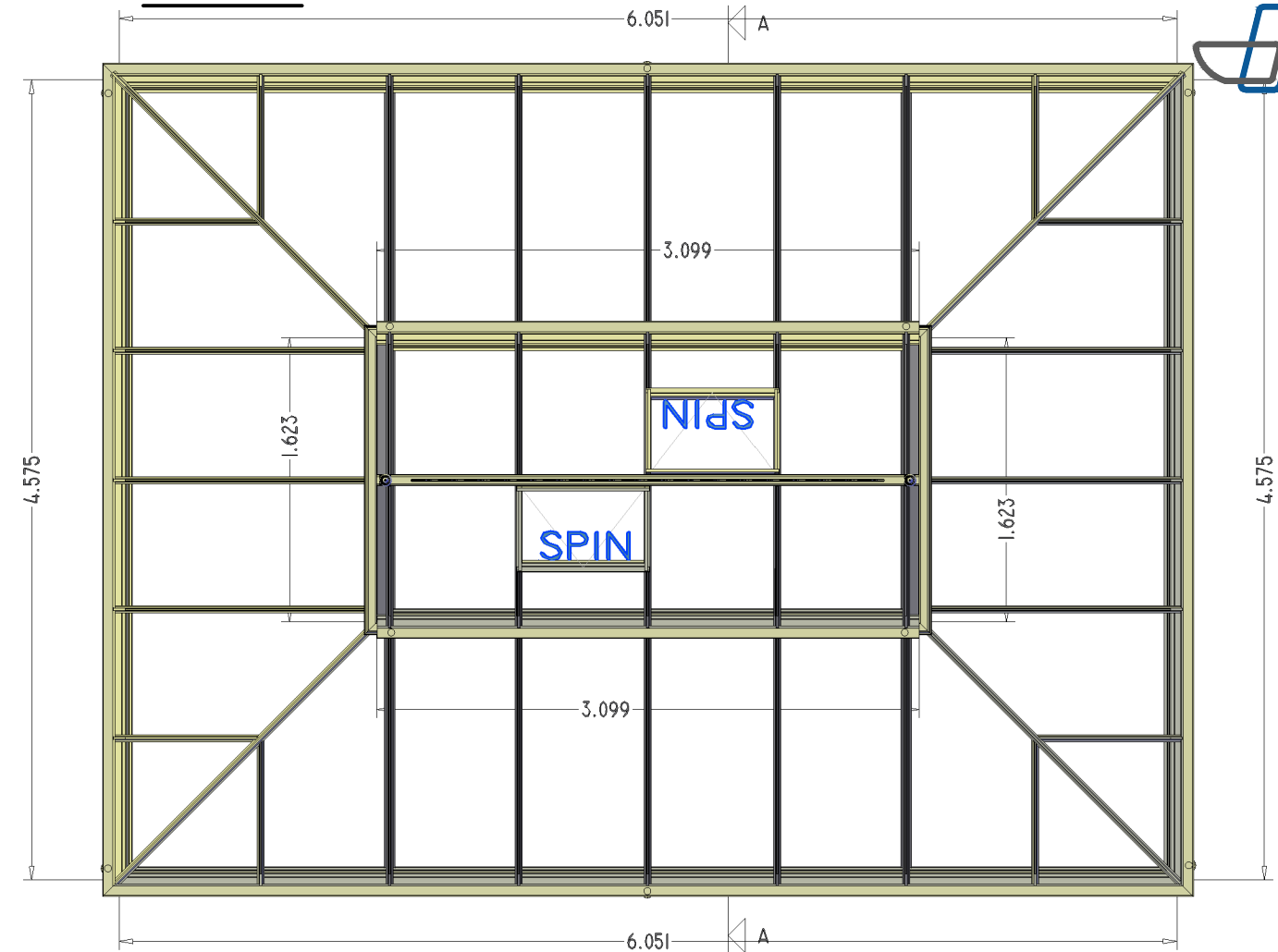
DACHPLAN
