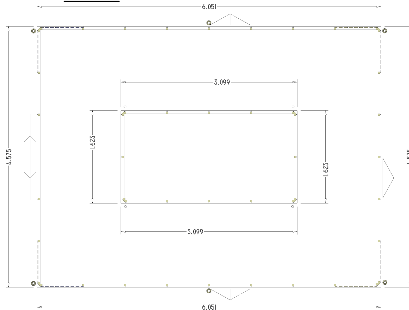
GRUNDRISS
